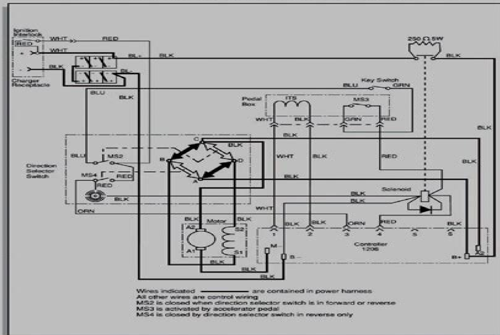
Fig. 19 Wiring Diagram
