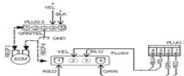
Fig. 13 - FE4A ECM / Plug Wiring Diagram
